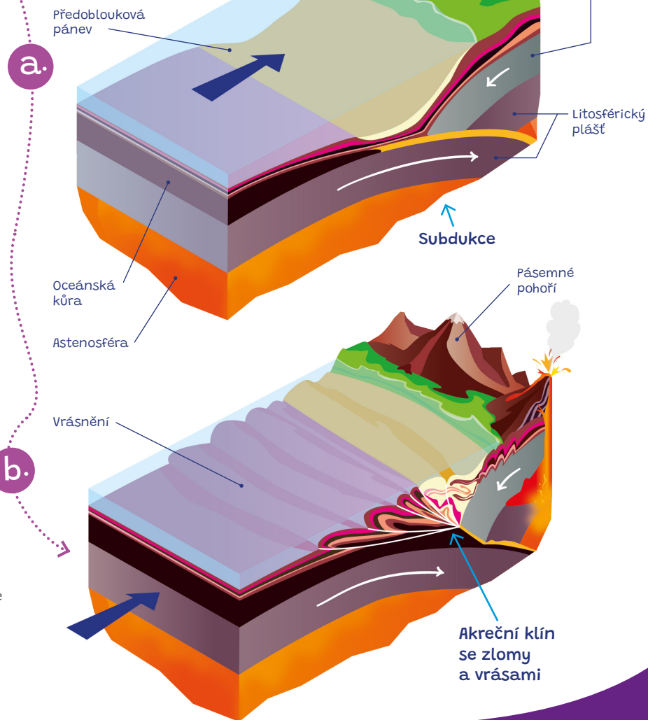
Obrázek 3 Schematický náčrt vzniku akrečního klínu v místě, kde se oceánská deska zasouvá pod kontinentální desku a během toho dochází ke stlačování svrchních horninových vrstev
