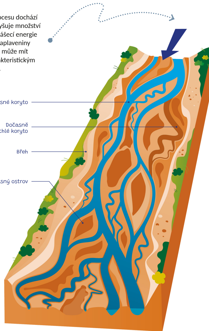
Obr. 3 Schematická ilustrace ukazující divočící řeku
